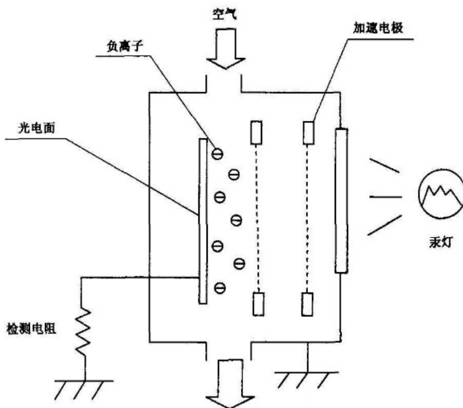
图 1 紫外电离原理图
