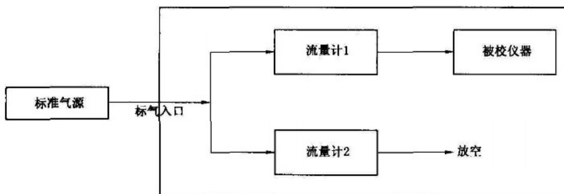
图2 流量控制器示意图
